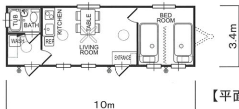
ランドブリッジ10m (本体全長10m x 幅3.4m)
